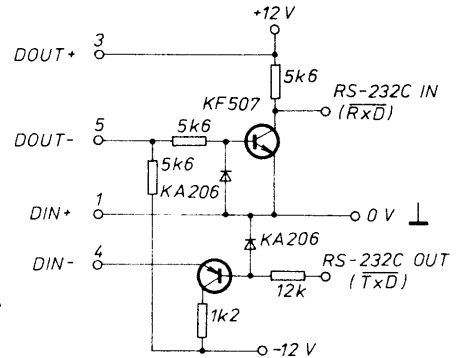
Obr. 6. Konvertor V.24 — PMD ↔ RS-232C
